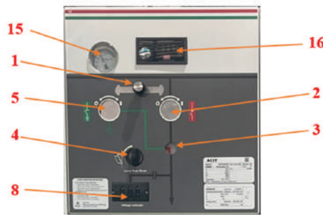
Mô-đun dao cắt tải | Load Break Switch module K
