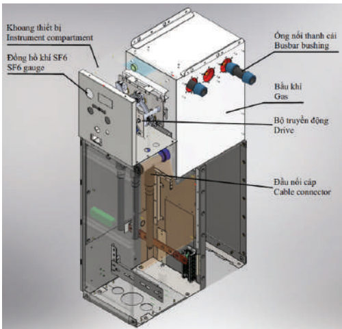
Mô-đun dao cắt tải | Load Break Switch module K
