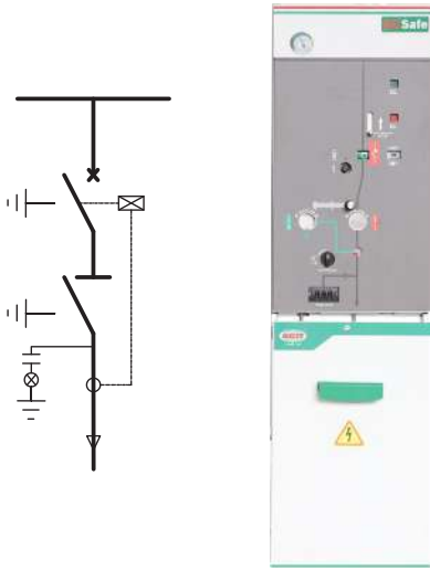
Chiều rộng / width: 375mm Chiều sâu / depth: 800mm Chiều cao / height: 1380mm
