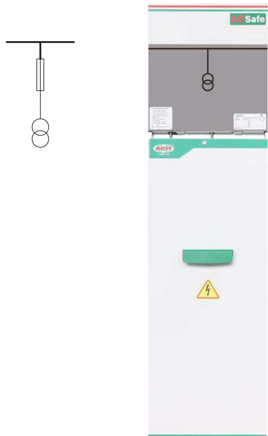
Chiều rộng / width: 800mm Chiều sâu / depth: 1000mm Chiều cao / height: 1380mm
