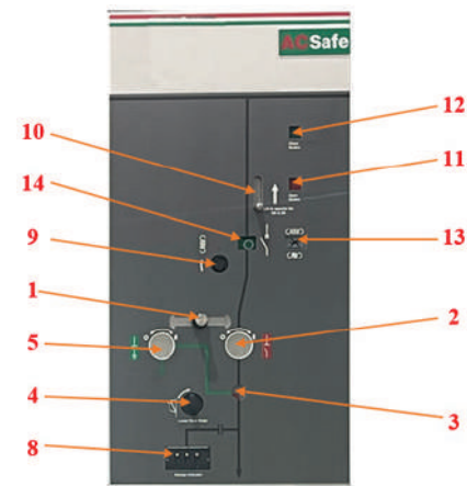
Mô-đun máy cắt | Circuit breaker module V
