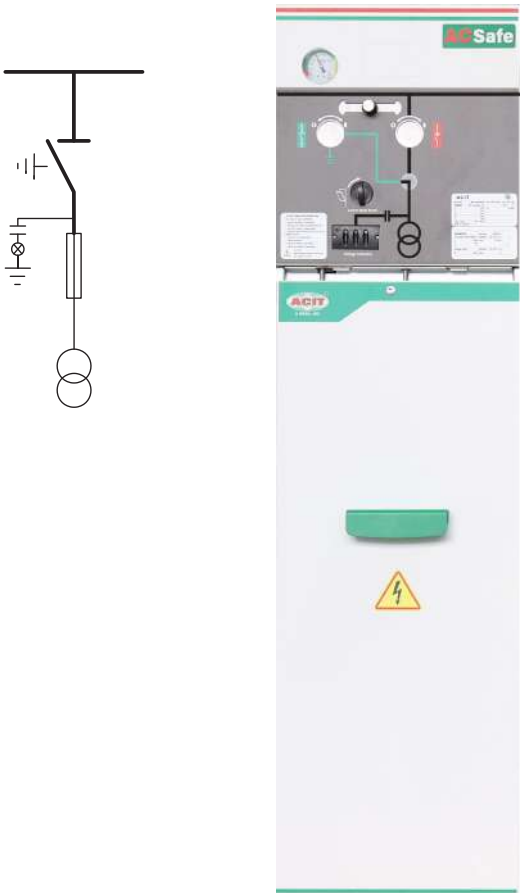
Chiều rộng / width: 600mm Chiều sâu / depth: 800mm Chiều cao / height: 1380mm
