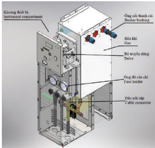
Mô-đun dao cắt tải-cầu chì | Load Break Switch Fuse module T
