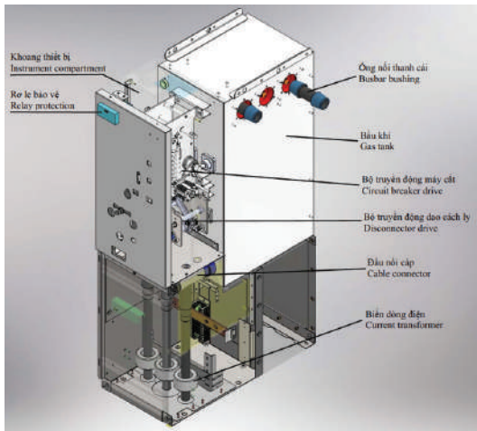
Mô-đun máy cắt | Circuit breaker module V
